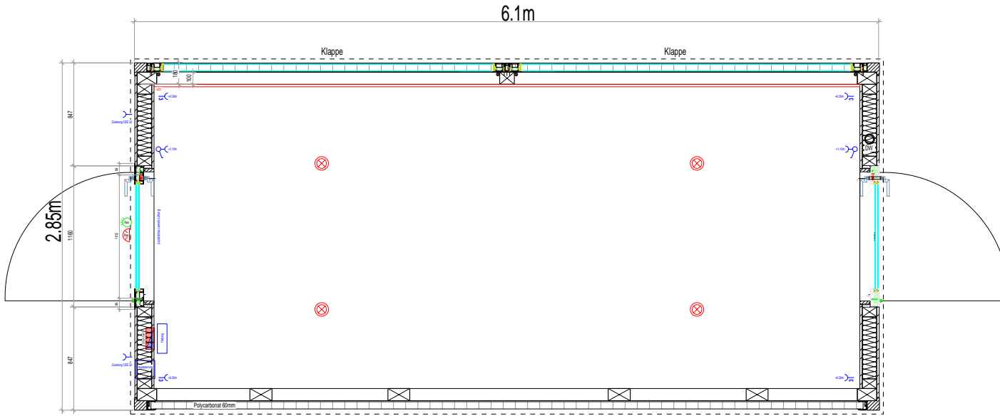
Grundriss
